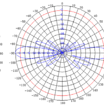
OD24M-9 E-Plane
