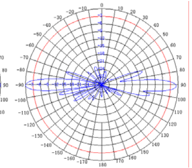
OD24M-12 E-Plane
