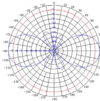
OD24M-5 E-Plane
