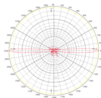
OD58M-12 E-Plane
