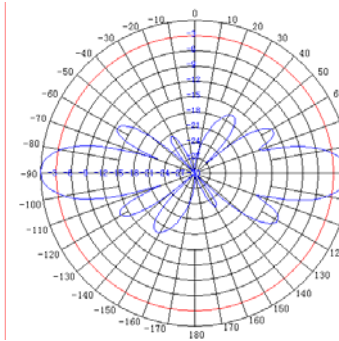
OD24M-7 E-Plane
