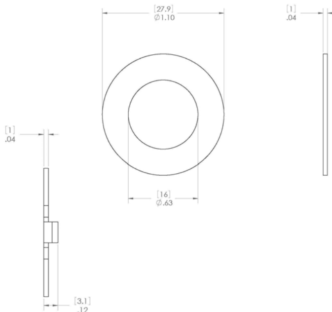
GASKET
