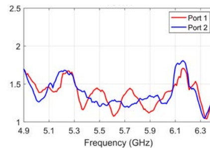
VSWR
